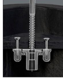
Sistema de pernos sin agarrotamiento Permite reemplazo de campo
